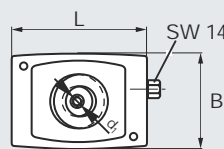
Avec trou fileté pour la fixation, Enfichable
